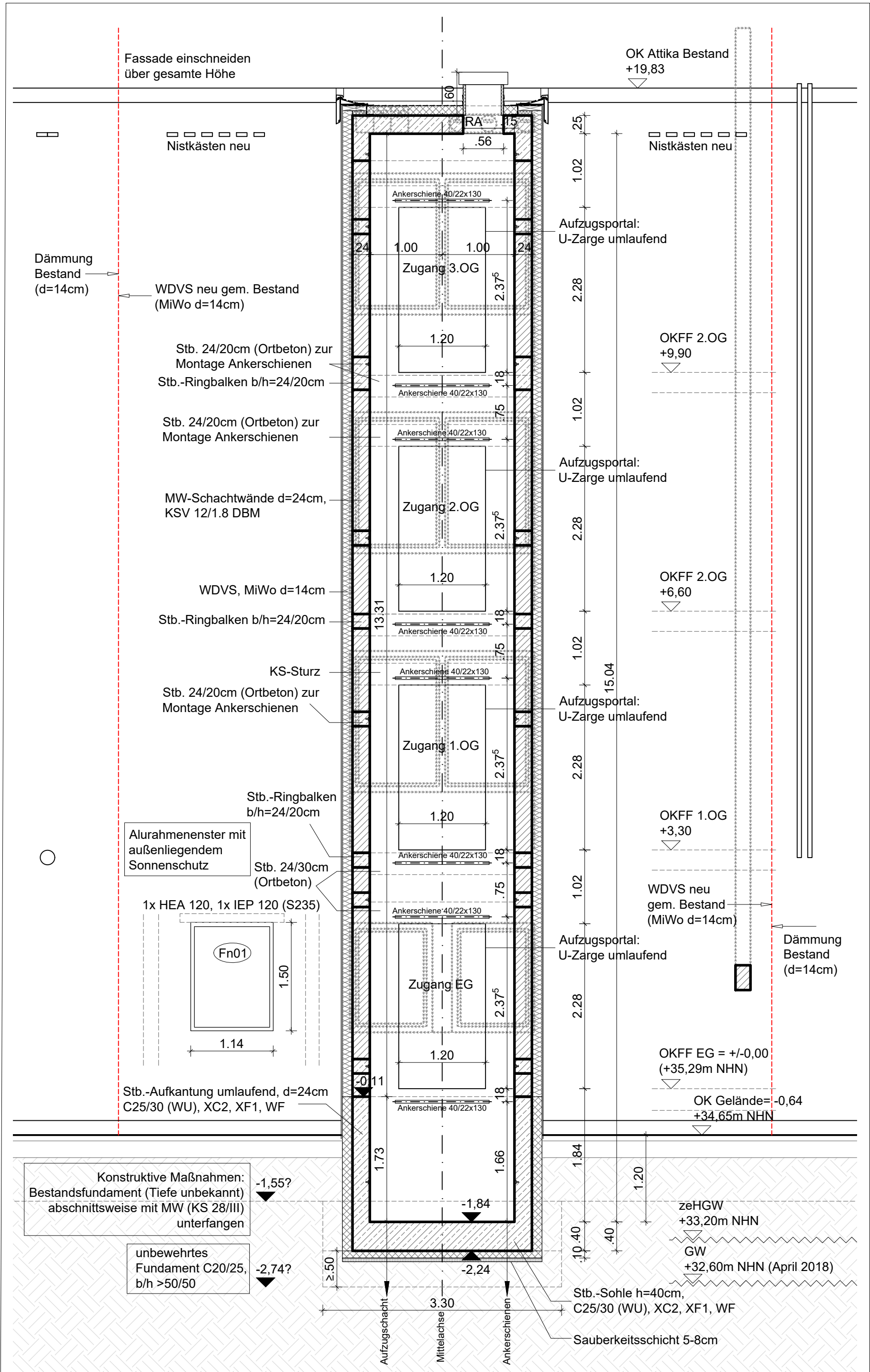
Schnitt BB / Aufzugsschacht
