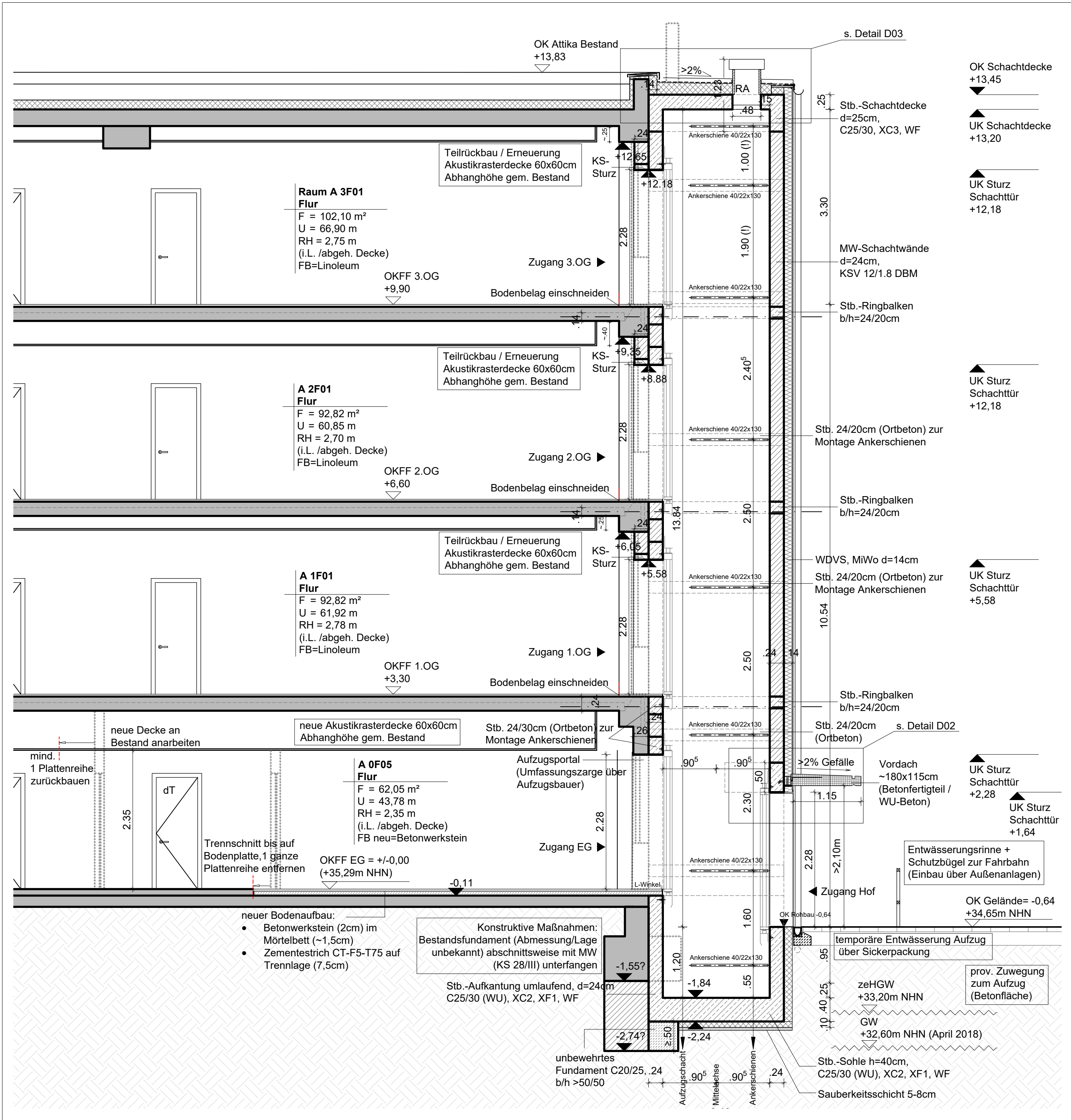
Schnitt AA / Aufzugsschacht
